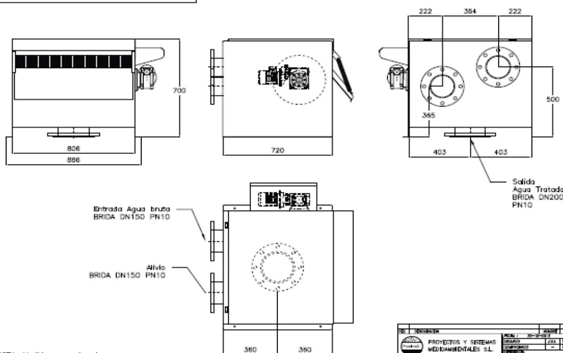
Rotofiltro Modelo 35-80
